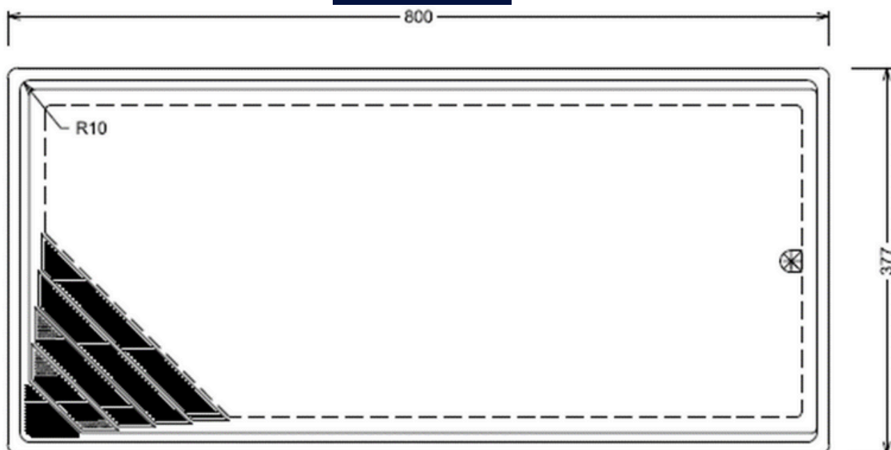
Grundriss
