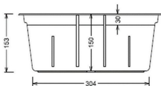
Ansicht Skimmerseite
