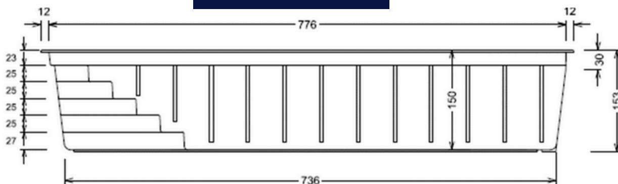
Seitenansicht
