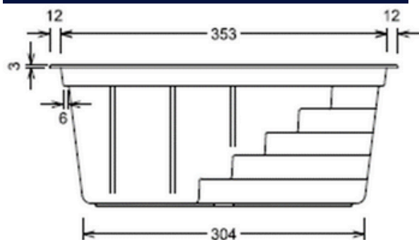
Ansicht Treppenseite
