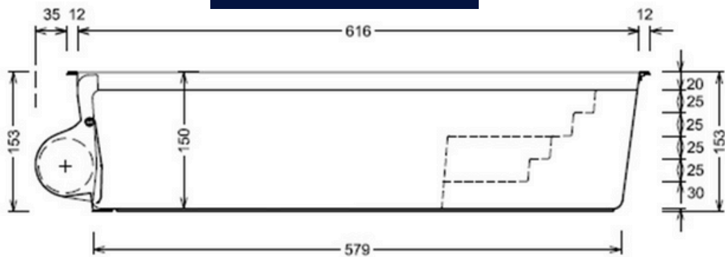
Seitenansicht
