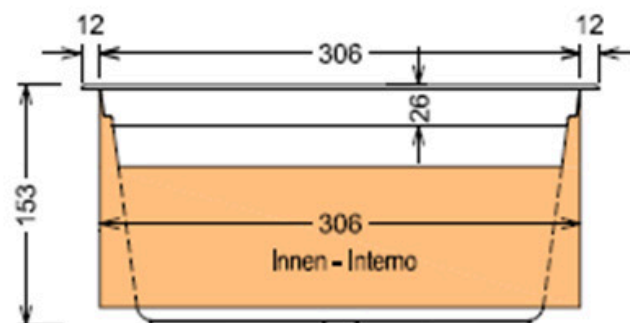
Ansicht Skimmerseite
