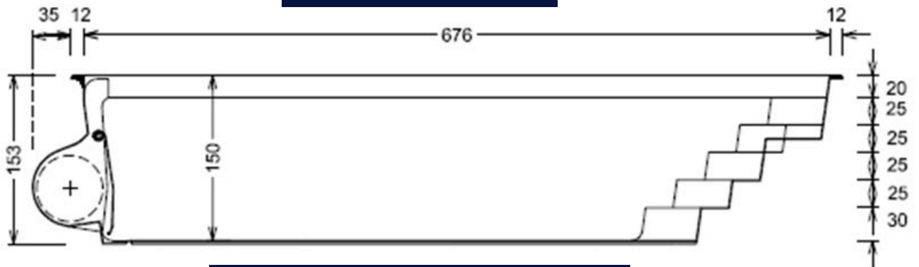
Ansicht Skimmerseite
