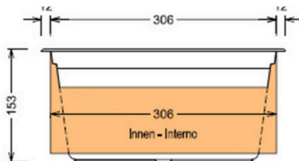
Ansicht Skimmerseite
